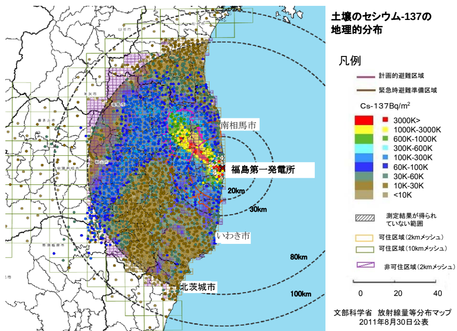
図7 セシウム-137の土壌濃度マップ
