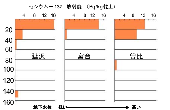
図 13 セシウムの土壌中での移動
